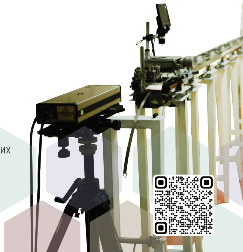
Уртын хэмжлийн анхдагч эталон | Иодоор тогтворжуулсан 633 нм долгионы урттай Гелий Неон лазер үүсгэгч
